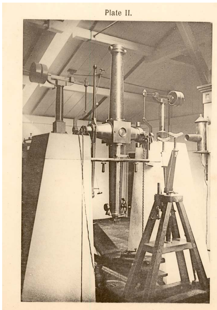
写真2 麻布時代のレプソルド子午儀の写真
