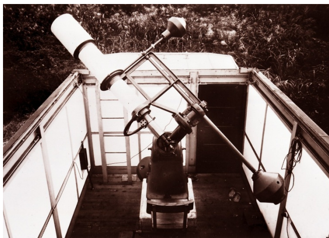
写真 1 口径 20cm の彗星捜索鏡
