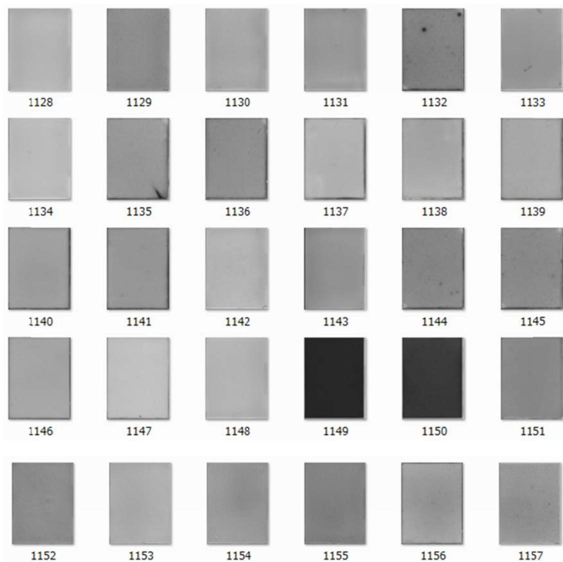
写真 2 ブラッシャー天体写真 BOX-002 のサムネイル
