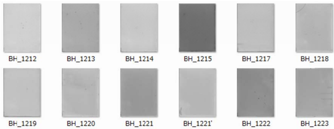
写真4 ブラッシャー天体写真 BOX-004 のサムネイル
