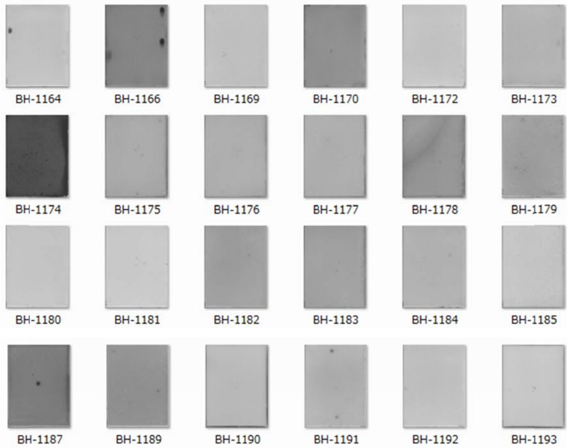
写真3 ブラッシャー天体写真 BOX-003 のサムネイル
