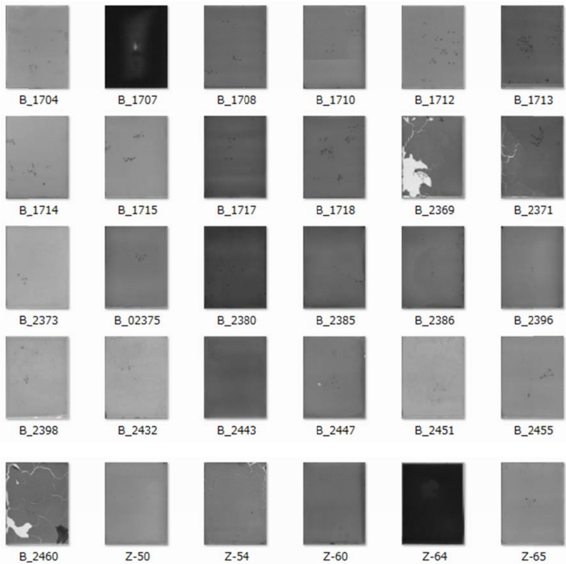
写真9 ブラッシャー天体写真 BOX-009 のサムネイル
