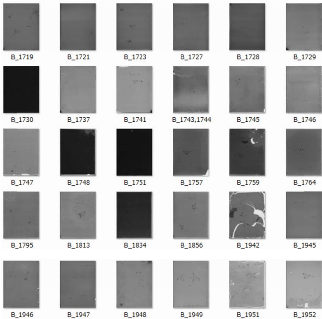
写真 10 ブラッシャー天体写真 BOX-010 のサムネイル
