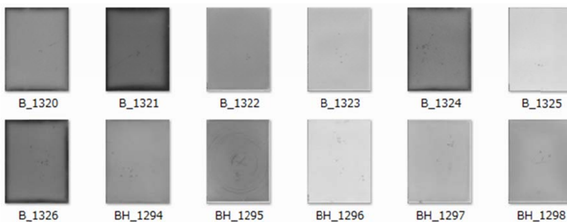
写真 6 ブラッシャー天体写真 BOX-006 のサムネイル
