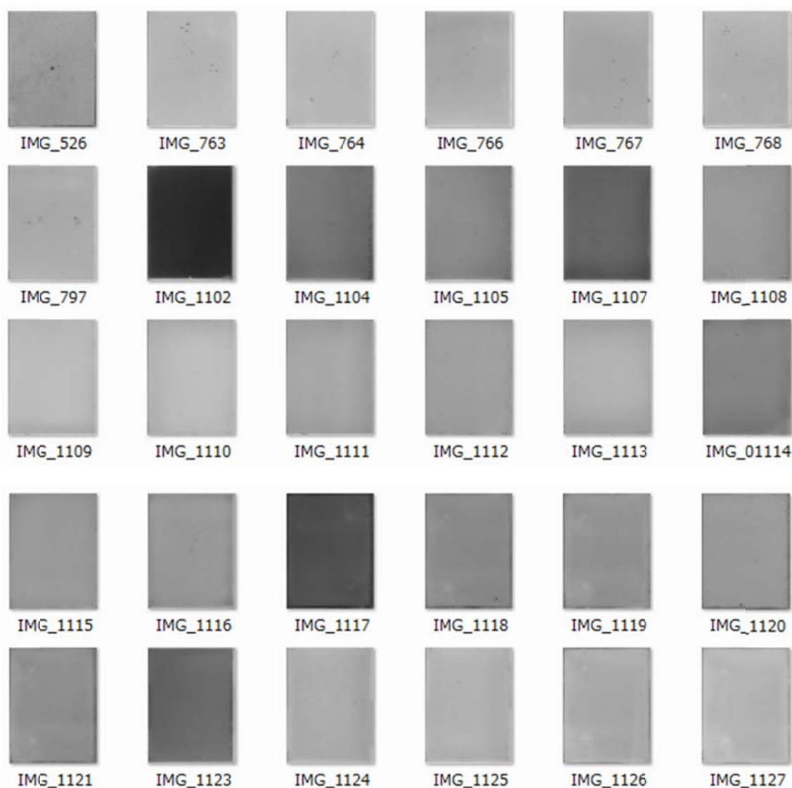
写真1 ブラッシャー天体写真 BOX-001 のサムネイル
