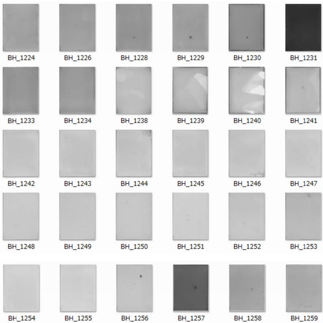
写真5 ブラッシャー天体写真 BOX-005 のサムネイル
