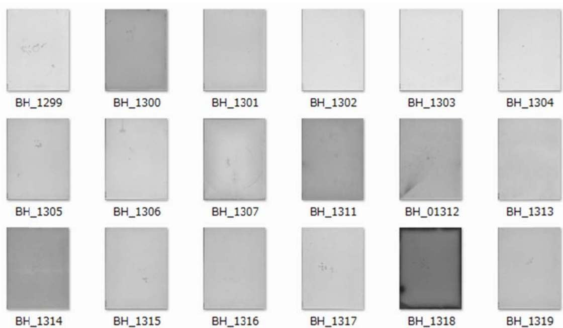
写真7 ブラッシャー天体写真 BOX-007 のサムネイル
