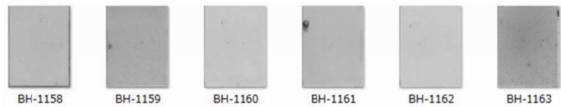
写真 2 ブラッシャー天体写真 BOX-002 のサムネイル
