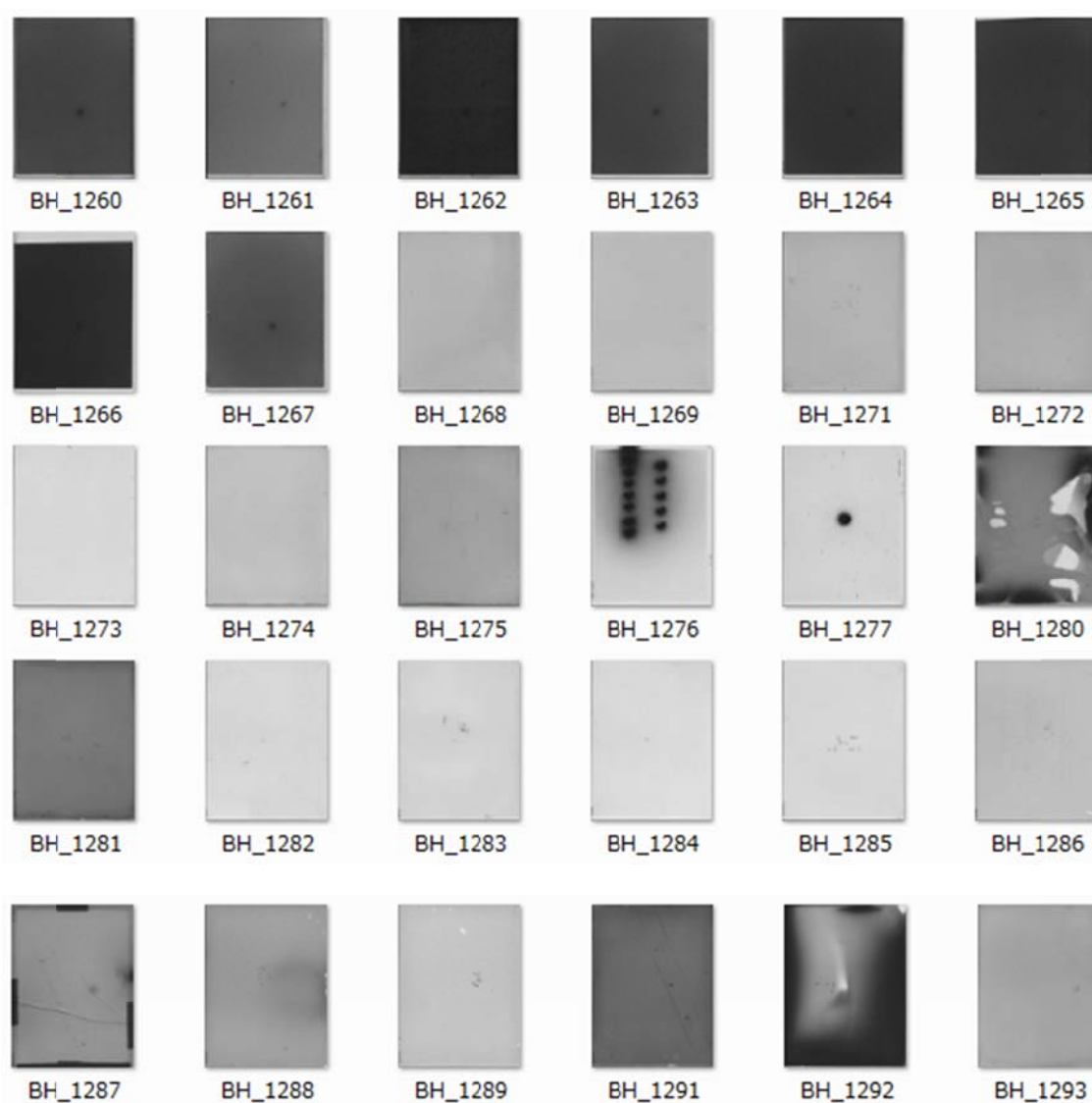
写真 6 ブラッシャー天体写真 BOX-006 のサムネイル
