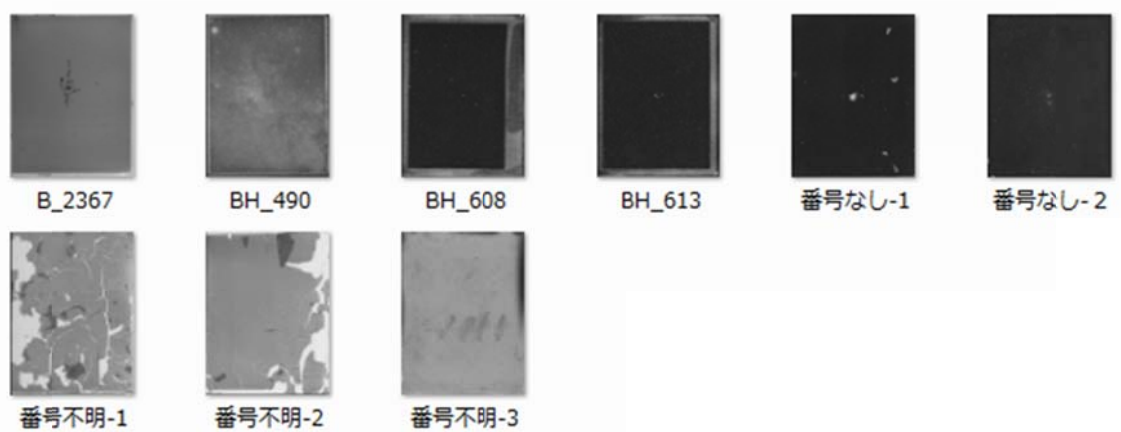
写真8 ブラッシャー天体写真 BOX-008 のサムネイル
