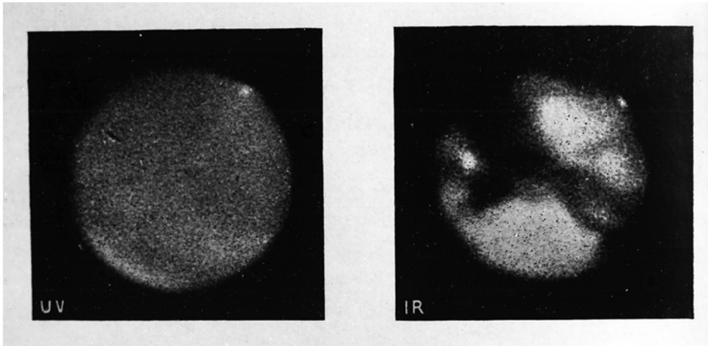
写真3 火星のUVとIRの比較
