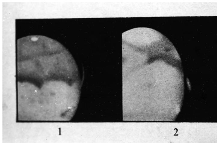
写真4 火星の写真 何を比較したものか不明
