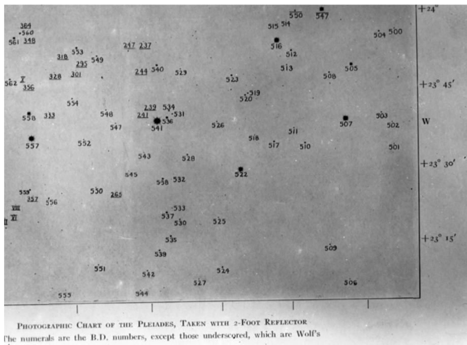
写真5 プレアデス星団のチャート
