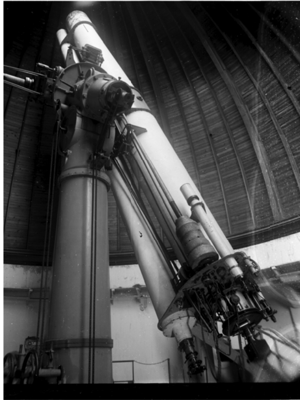
写真4 光電受光機を取りつけた26”屈折望遠鏡 他に2枚の写真があり、写真5がプレアデス星団のチャートで、「PHOTOGRAPHIC CHART OF THE PLEIADES, TAKEN WITH 2-FOOT REFLECTOR」と書かれている。
