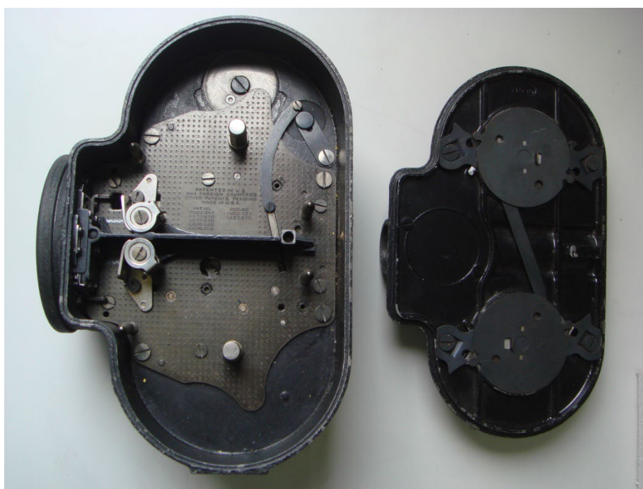
写真 4 フィルムを装填する蓋を外したところ
