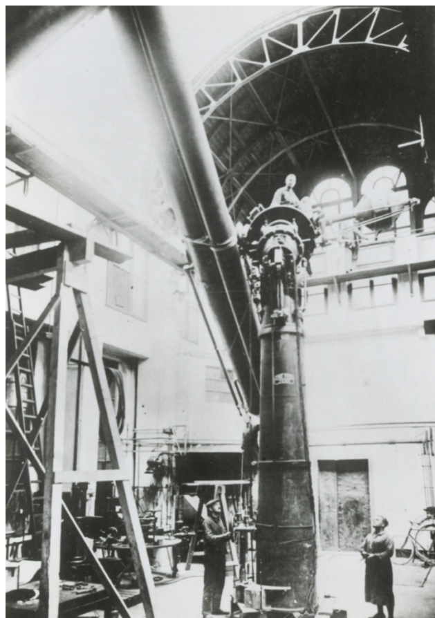
写真3 ドイツ・ツアイス社での検収の様子
