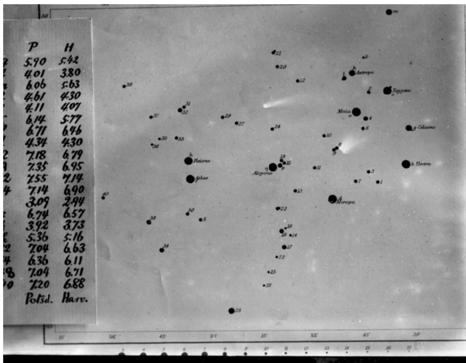
写真6 プレアデス星団の星野-2
