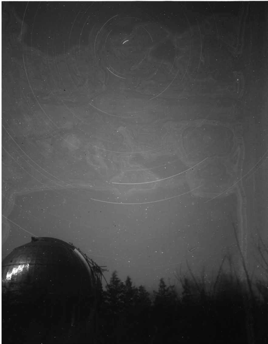
写真4 26”望遠鏡ドームを背にした周極星野
