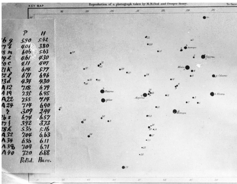
写真5 プレアデス星団の星野
