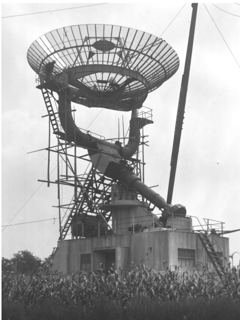
写真 5 建設中の 10m パラボラアンテナ
