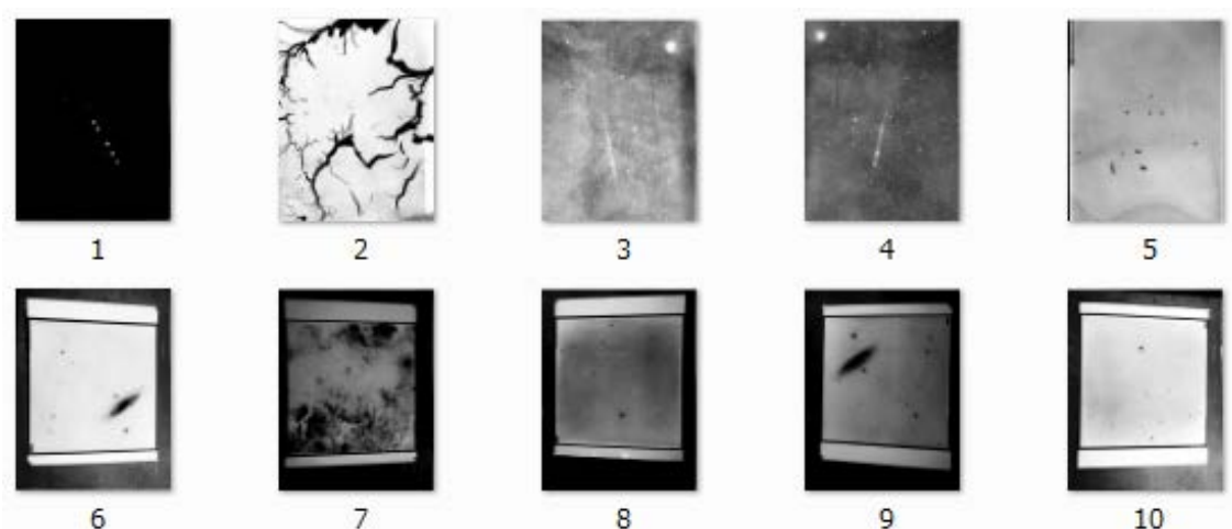
写真2 48” Schmidt 写真10枚のサムネイル
