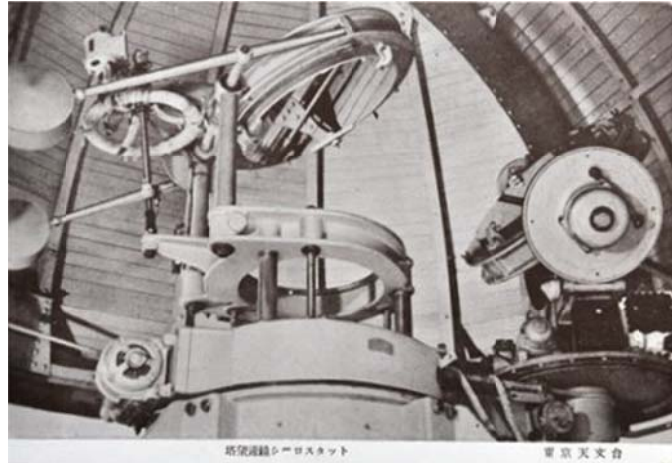
写真9 太陽塔望遠鏡シーロスタット
