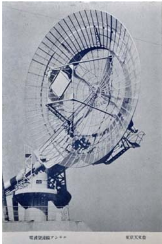
写真12 10m 太陽電波望遠鏡
