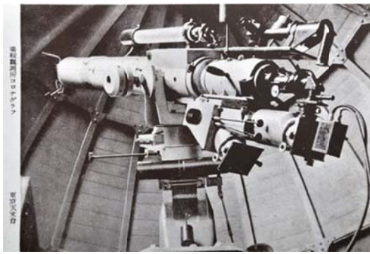
写真10 乗鞍コロナ観測所 10 cm コロナグラフ
