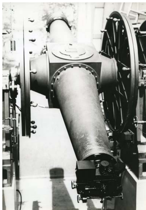
写真4 ゴーチェ子午環
